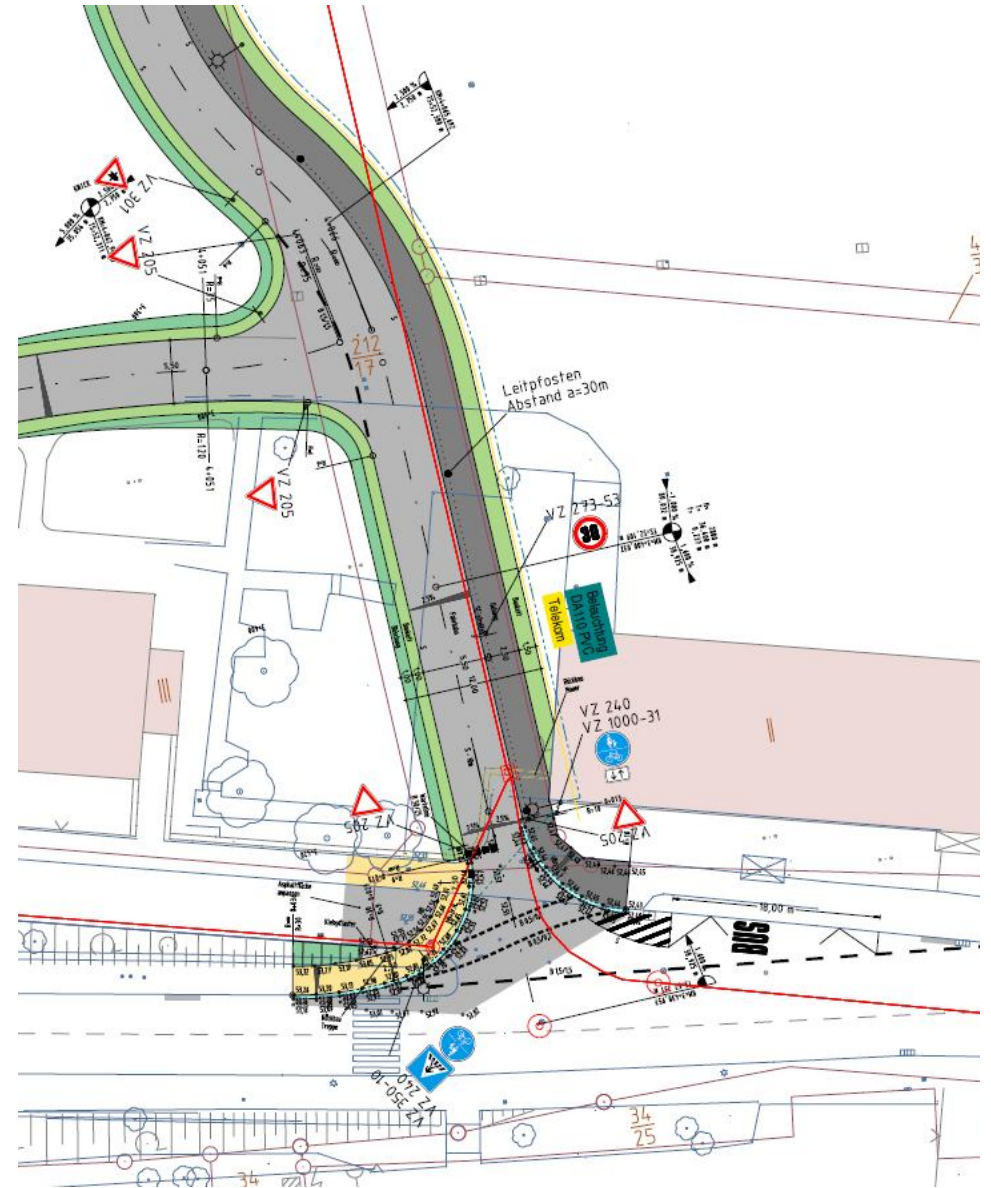
Ersatzerschließungsstraße mit Anschluss an Wunstorfer Straße und Verkehrsbeschilderung
